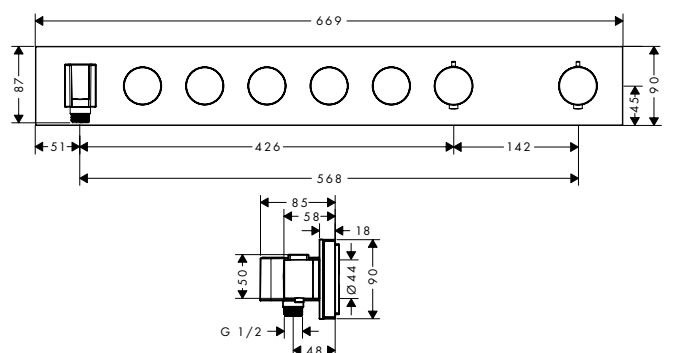
Module thermostatique Select encastré 670/900 avec 5 fonctions
