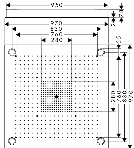
ShowerHeaven 970/970 avec éclairage
