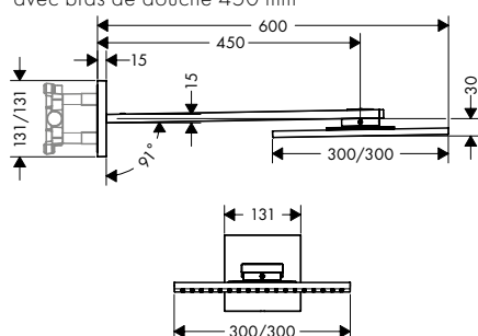
Douche de tête 300/300 mm 2jet avec bras de douche 450 mm
