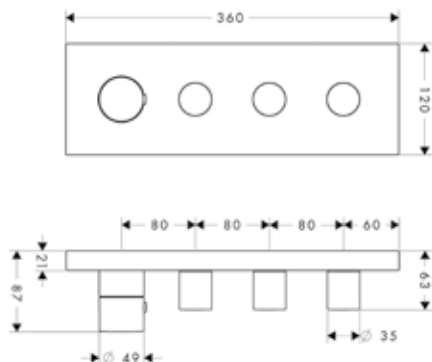
Module thermostatique encastré 360/120 avec 3 fonctions
