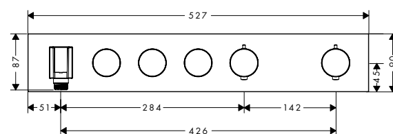
Module thermostatique encastré Select 530/90 pour 3 fonctions
