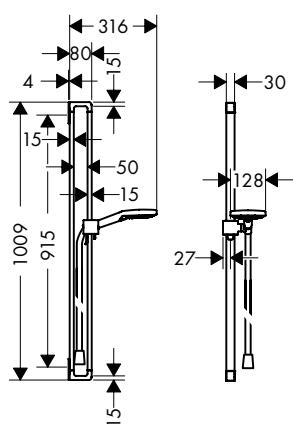
Set de douche 0,90 m avec douchette 120 3jet
