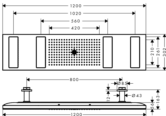
ShowerHeaven 1200/300 4jet avec éclairage 2700 K
