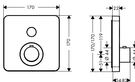
Thermostatique ShowerSelect SoftCube encastré pour 1 fonction
